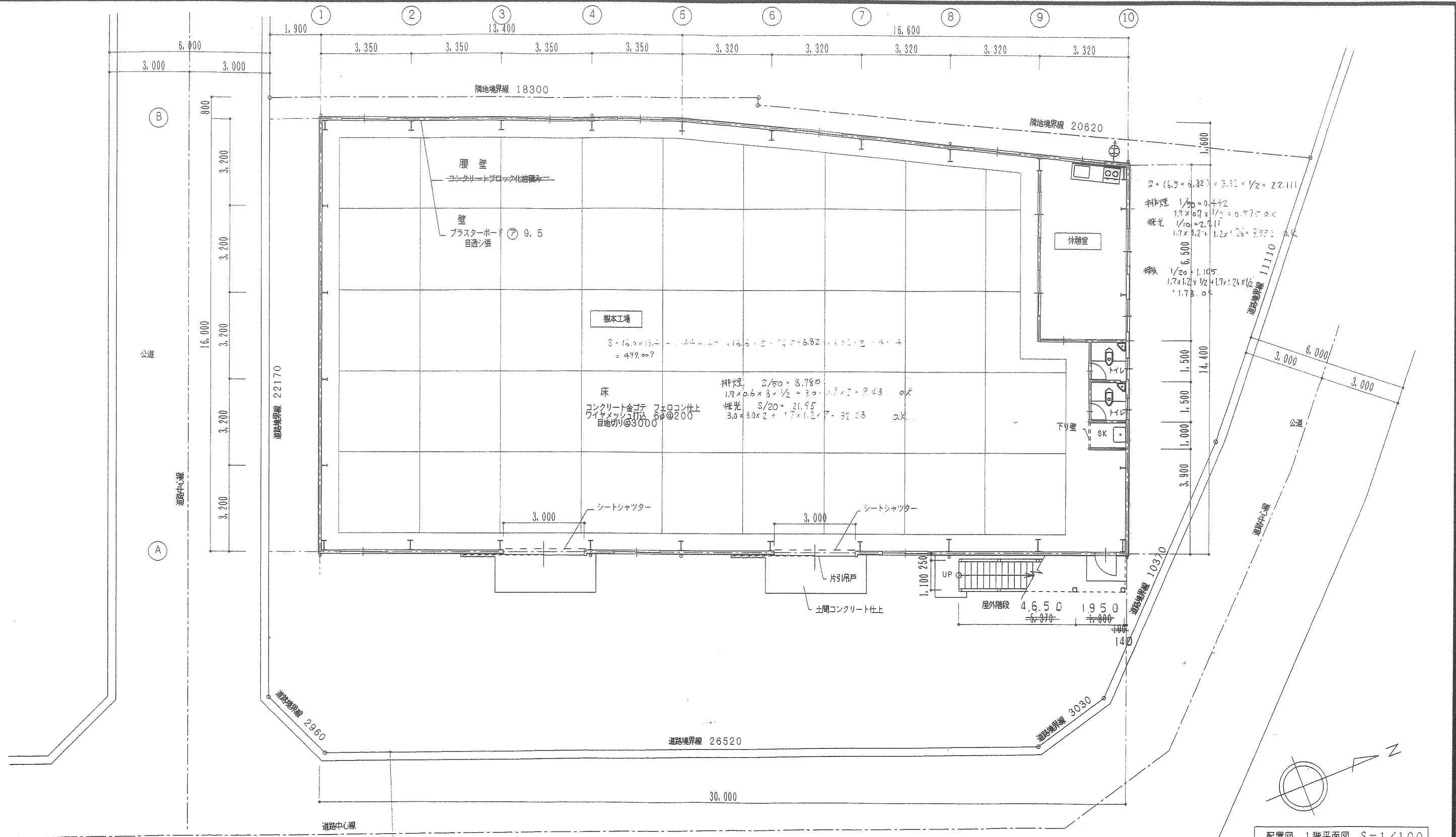
配置図、1階平面図 S=1/100
